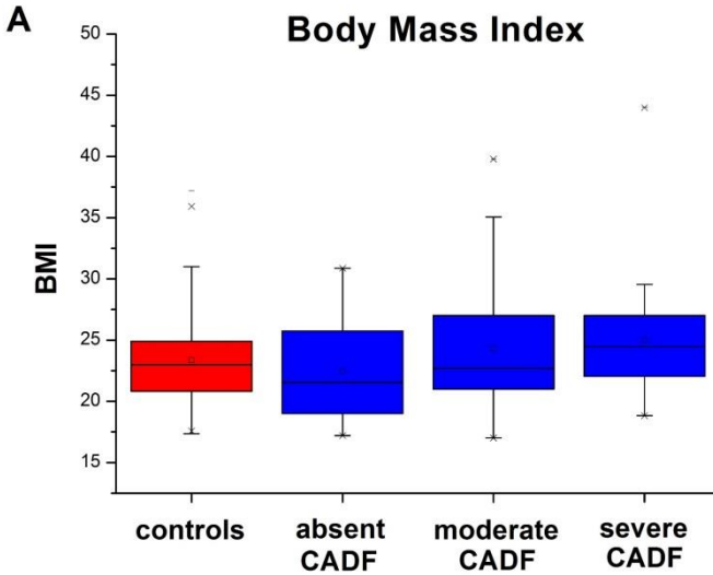
Abbildung 4: Body Mass
